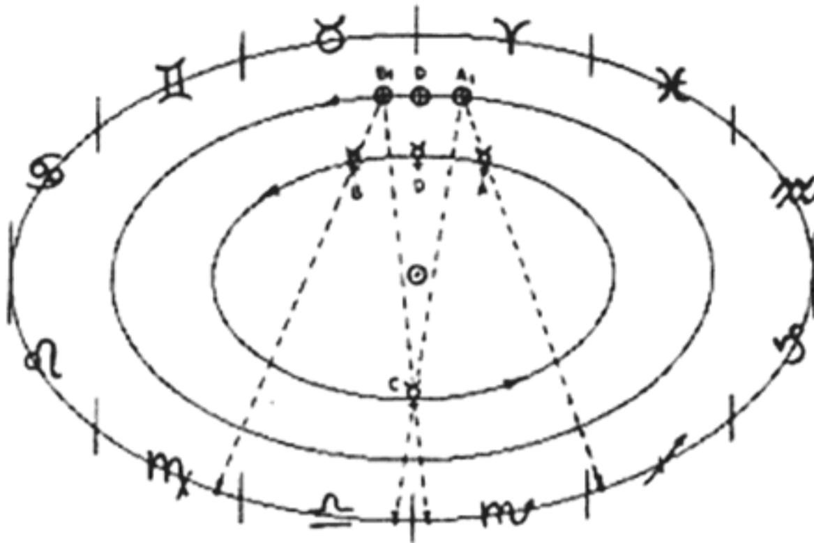
Figura 2: Movimiento retrógrado de un planeta interior
